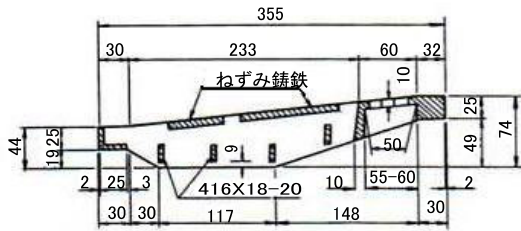
都型汚水ますふた
